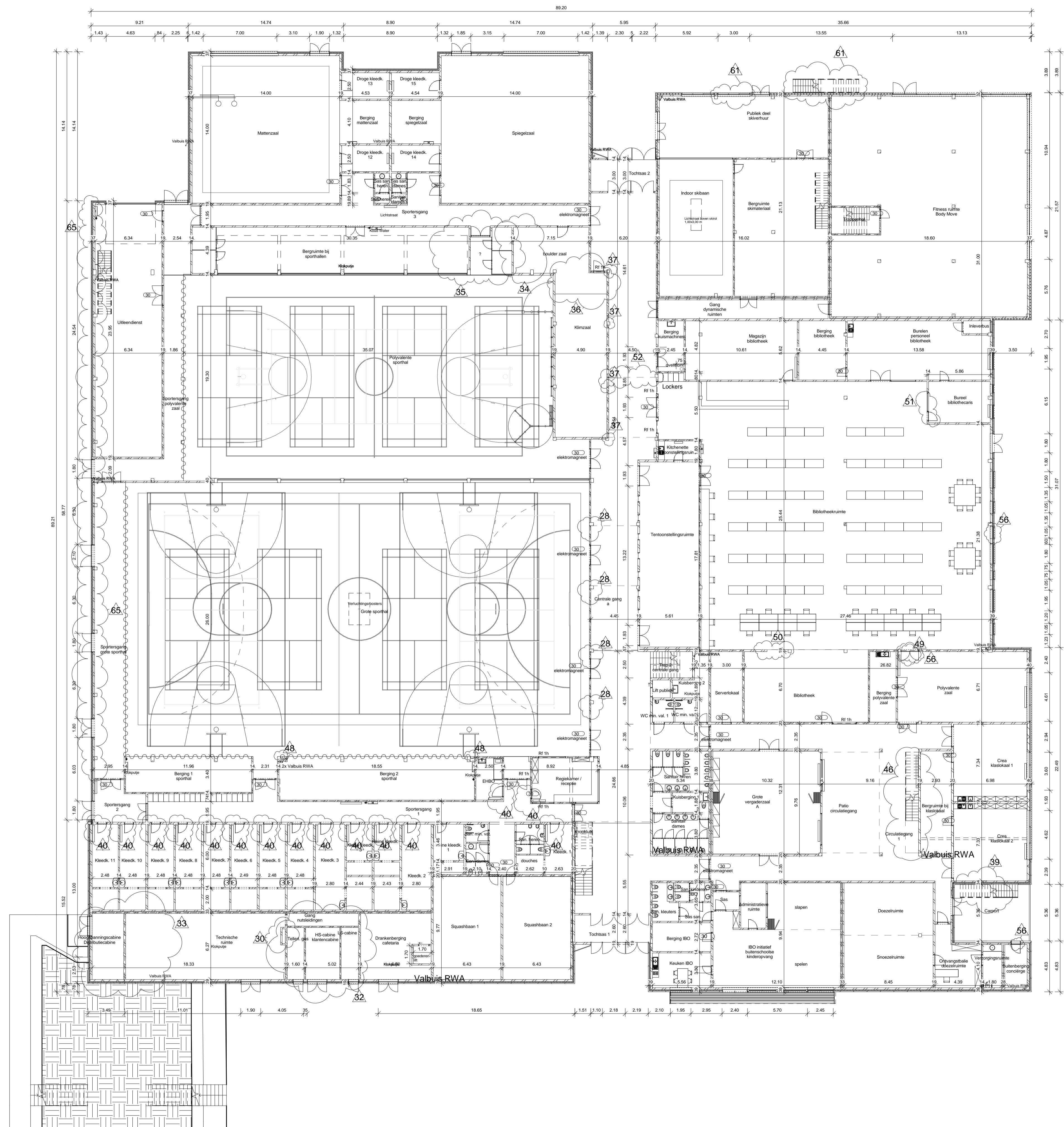
1 00 Gelijkvloers 1/200 1 : 200
